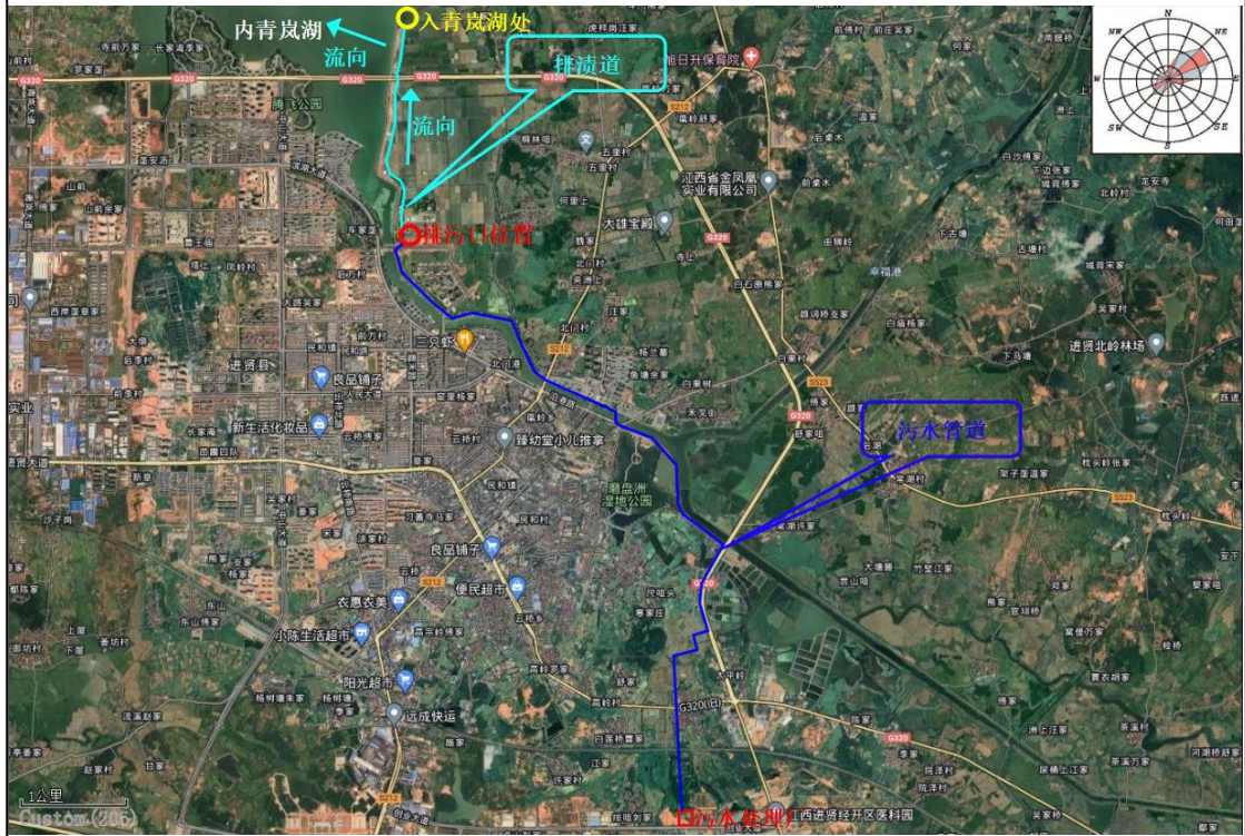
排污单位-排污管线-入河排污口-接纳水体排污走向图:
